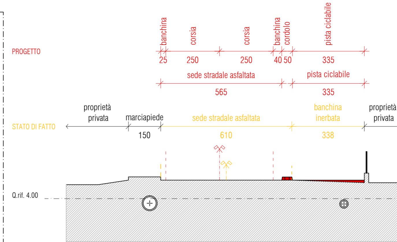
SEZIONE 3-3 QUOTATA CON INDICAZIONI DI STERZO/RIPORTO Scala 1:100
