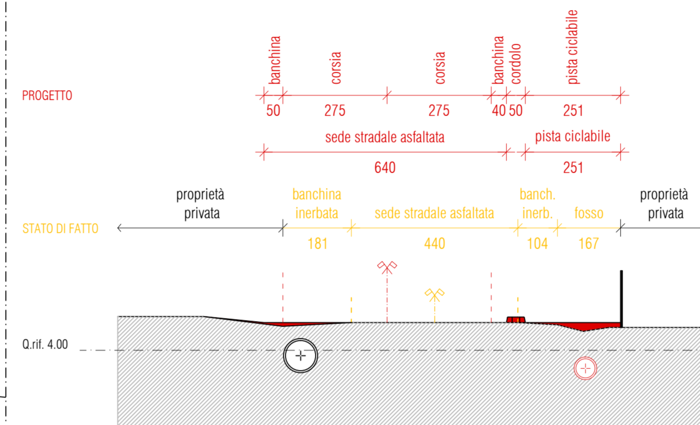
SEZIONE 4-4 QUOTATA CON INDICAZIONI DI STERZO/RIPORTO Scala 1:100
