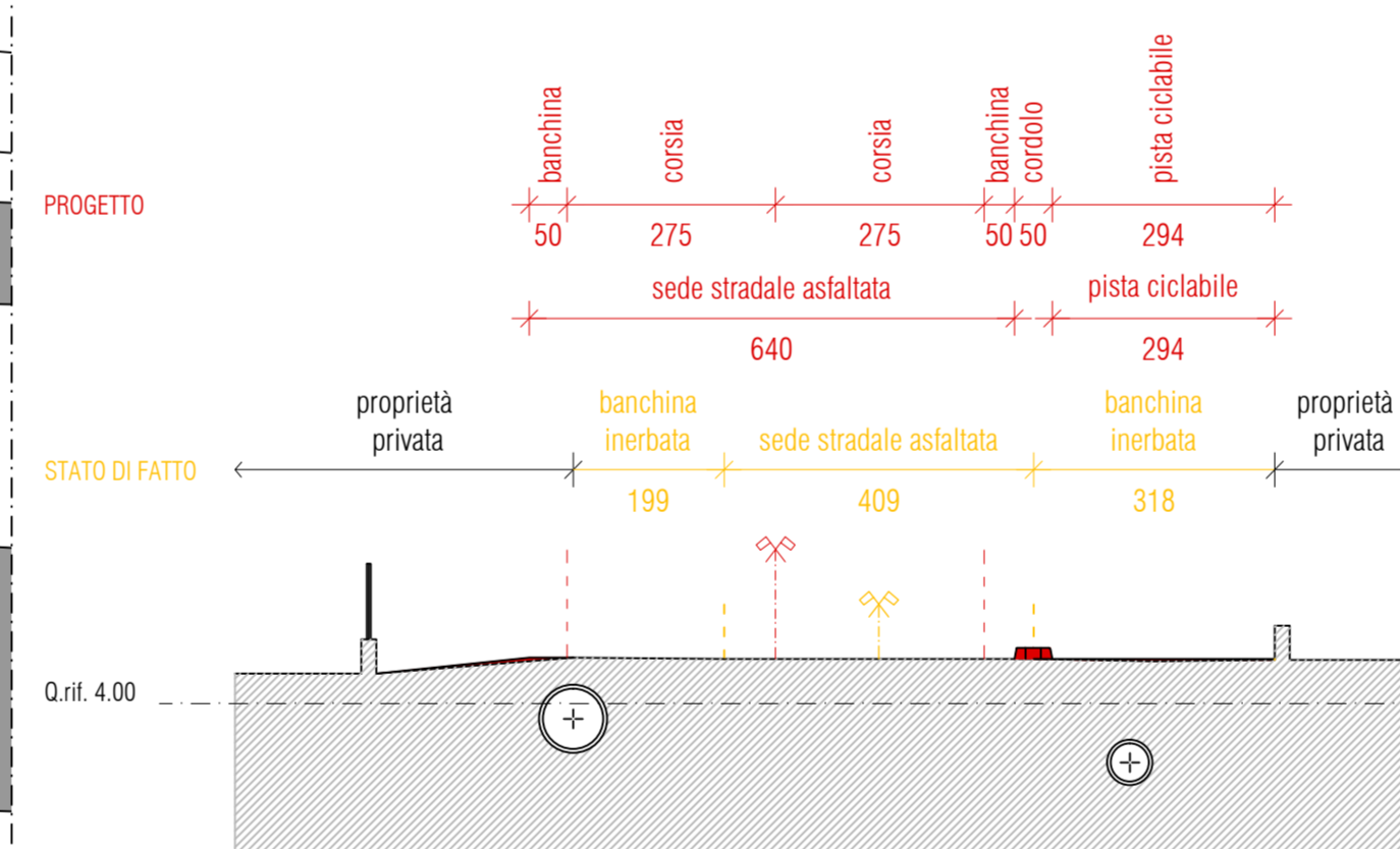
SEZIONE 5-5 QUOTATA CON INDICAZIONI DI STERZO/RIPORTO Scala 1:100
