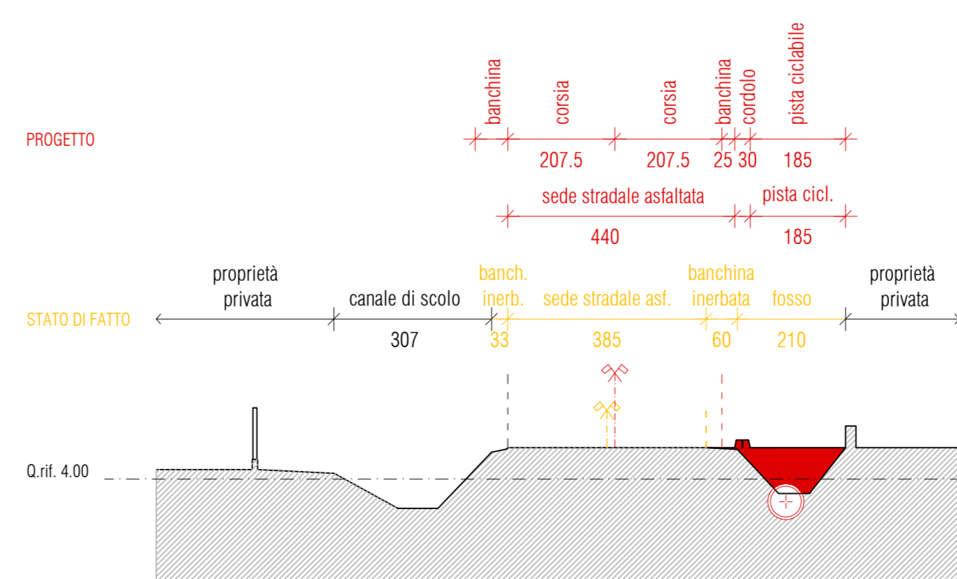
SEZIONE 8-8 QUOTATA CON INDICAZIONI DI STERZO/RIPORTO Scala 1:100
