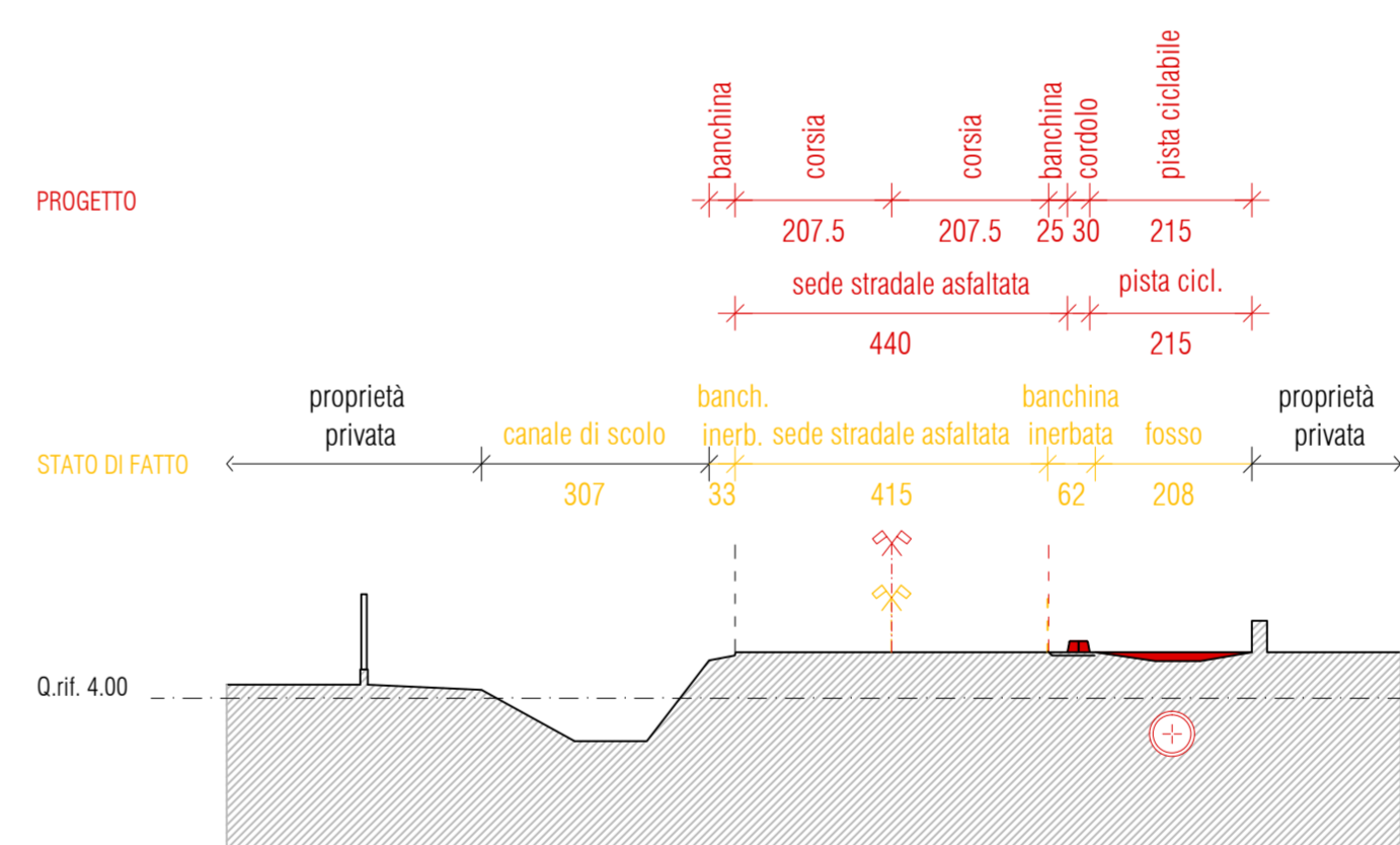
SEZIONE 7-7 QUOTATA CON INDICAZIONI DI STERZO/RIPORTO Scala 1:100
