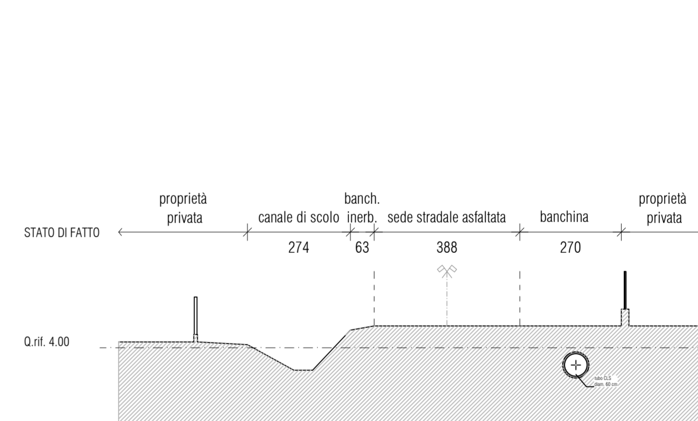
SEZIONE FINE TRATTO DI INTERVENTO QUOTATA Scala 1:100
