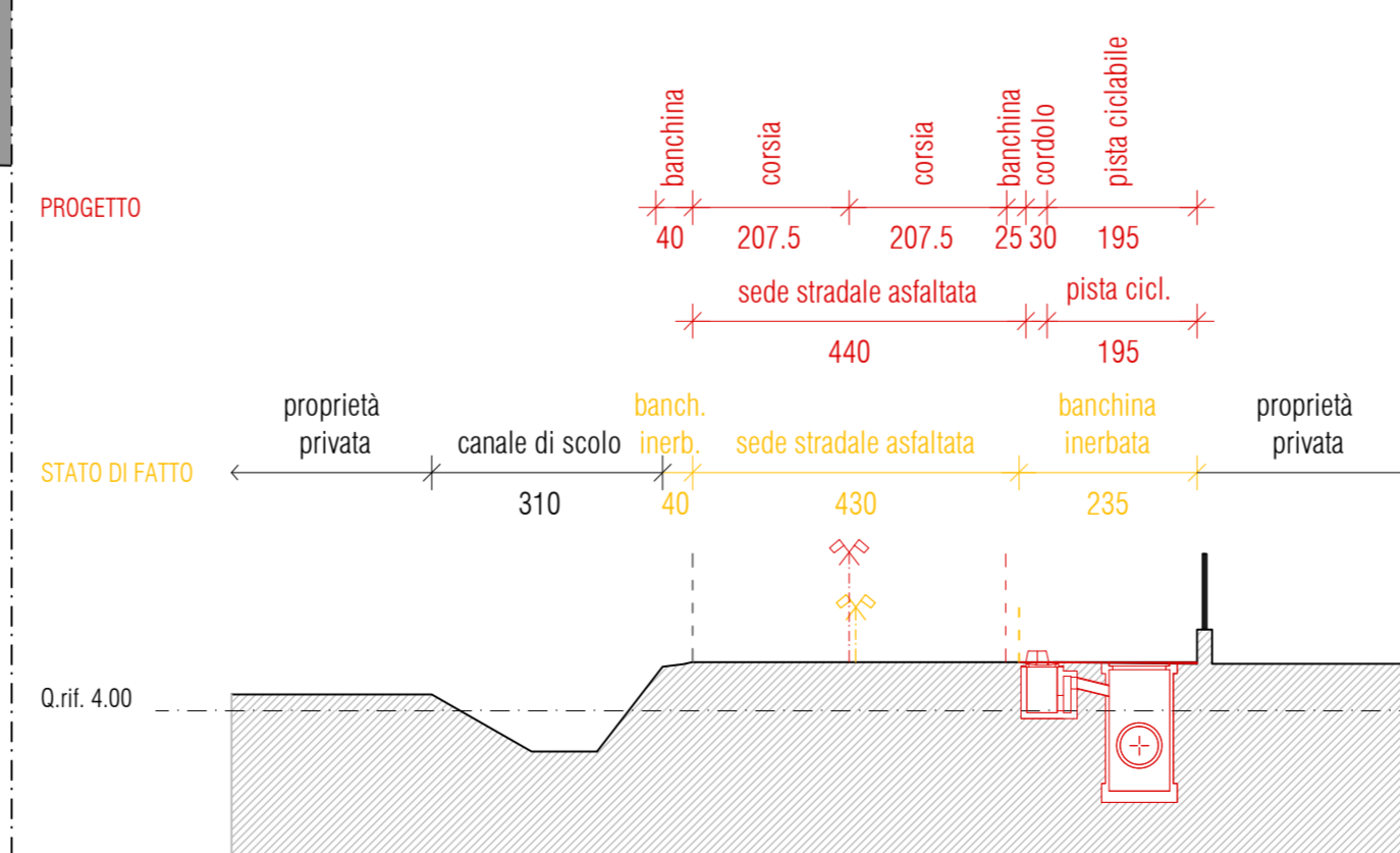
SEZIONE 6-6 QUOTATA CON INDICAZIONI DI STERZO/RIPORTO Scala 1:100
